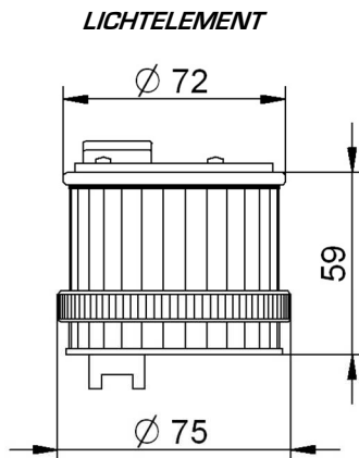
LICHTELEMENT
