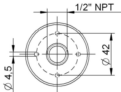
TSZ 8600
