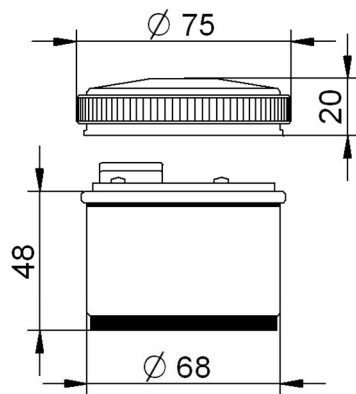
TSZ 8600
