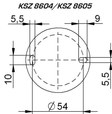
KSZ 8604/KSZ 8605
