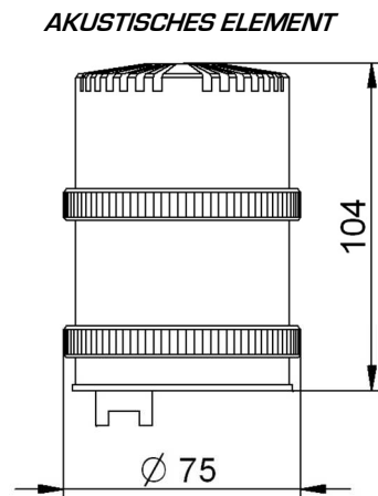
AKUSTISCHES ELEMENT
